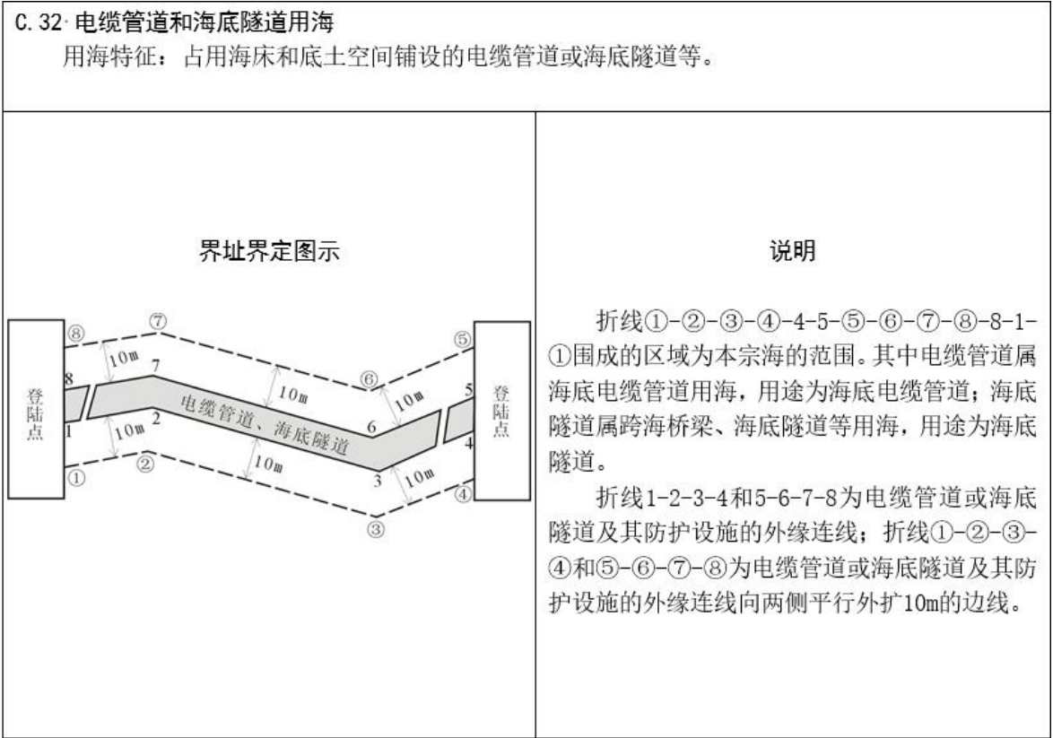
图 7.5.2-1 电缆管道和海底隧道用海宗海界址界定示例
