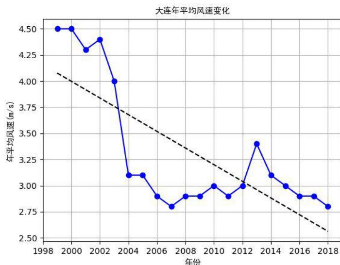
图 3.2.1-6 大连（1999-2018）年平均风速
