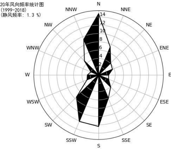
图 3.2.1-5 大连风向玫瑰图
